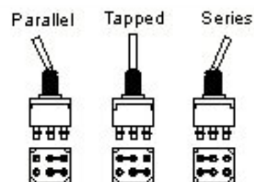
ON-ON-ON type Mini toggle switch
